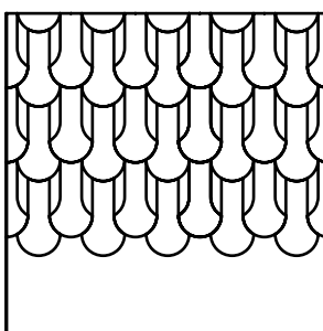
1/2 GRA EC 2 D / 17 ÉCAILLE 2 DEMI 1200 X 1200 mm
